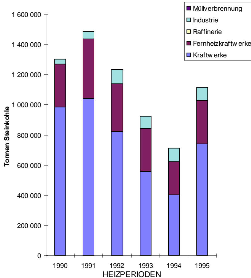
Abb. 3.1.1.1: Steinkohleverbrauch in DKA > 50 MW
