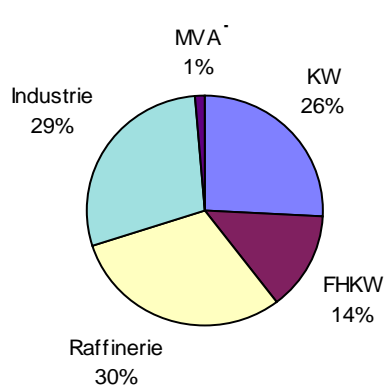
Abb. 3.1.1.25: NO x -Emissionen der DKA > 50 MW in der Heizperiode 1995
