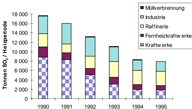
Abb. 3.1.1.19: SO 2 -Emissionen der DKA > 50 MW
