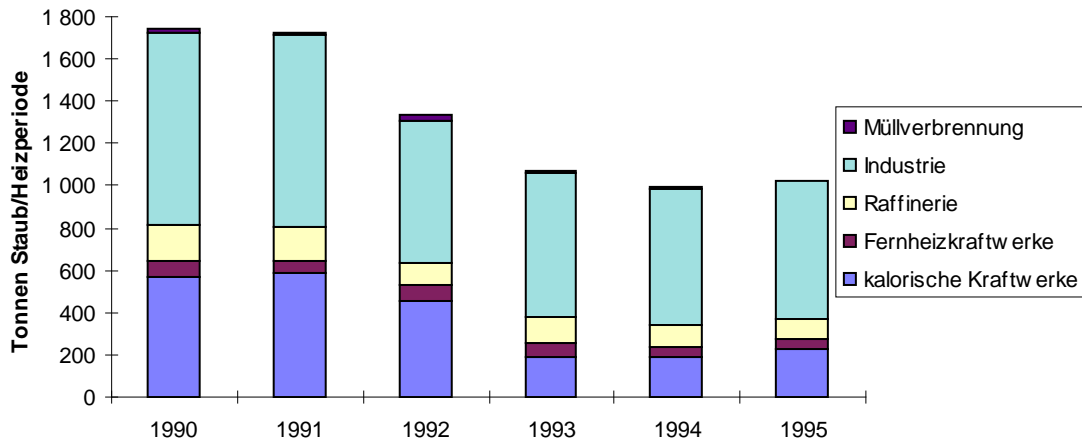
Abb. 1.3: Staub-Emissionen der DKA in Österreich
