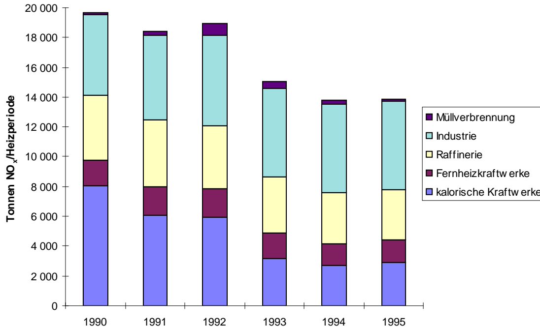
Abb. 1.2: NO x -Emissionen der DKA in Österreich
