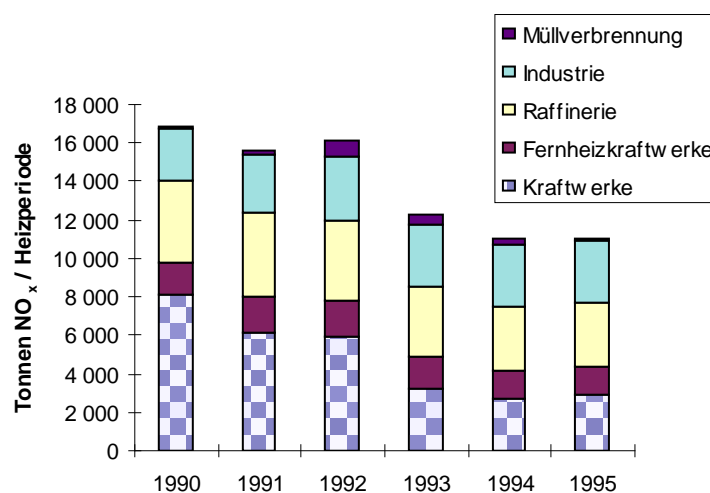
Abb. 3.1.1.20: NO x -Emissionen der DKA > 50 MW
