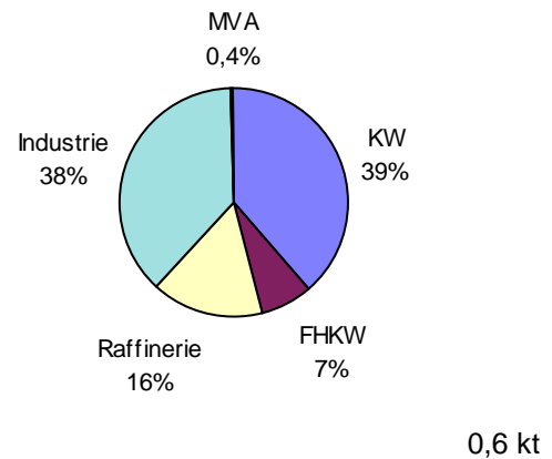
Abb. 3.1.1.27: Staub-Emissionen der DKA > 50 MW in der Heizperiode 1995
