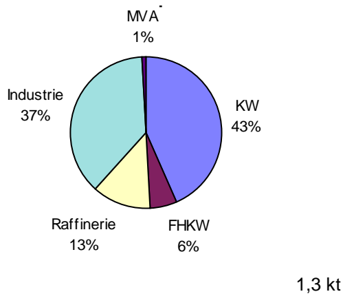
Abb. 3.1.1.26: Staub-Emissionen der DKA > 50 MW in der Heizperiode 1990
