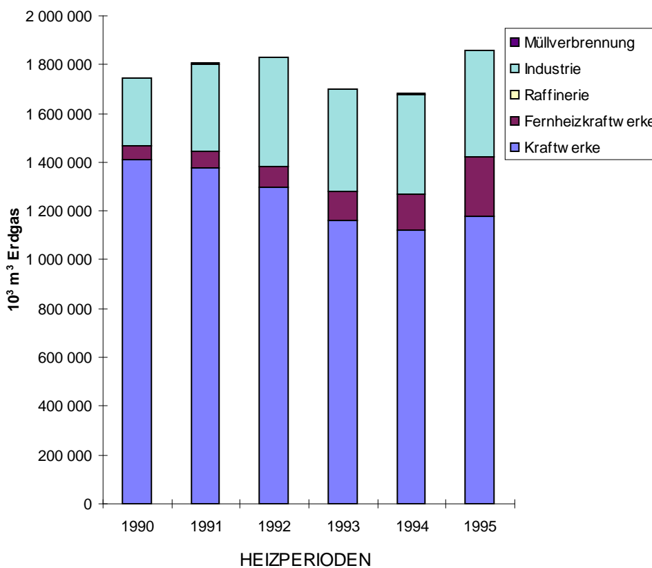
Abb. 3.1.1.3: Erdgasverbrauch in DKA > 50 MW
